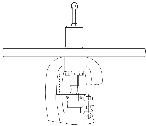
Рис. 2: \geq DN 250 со шкалой хода
