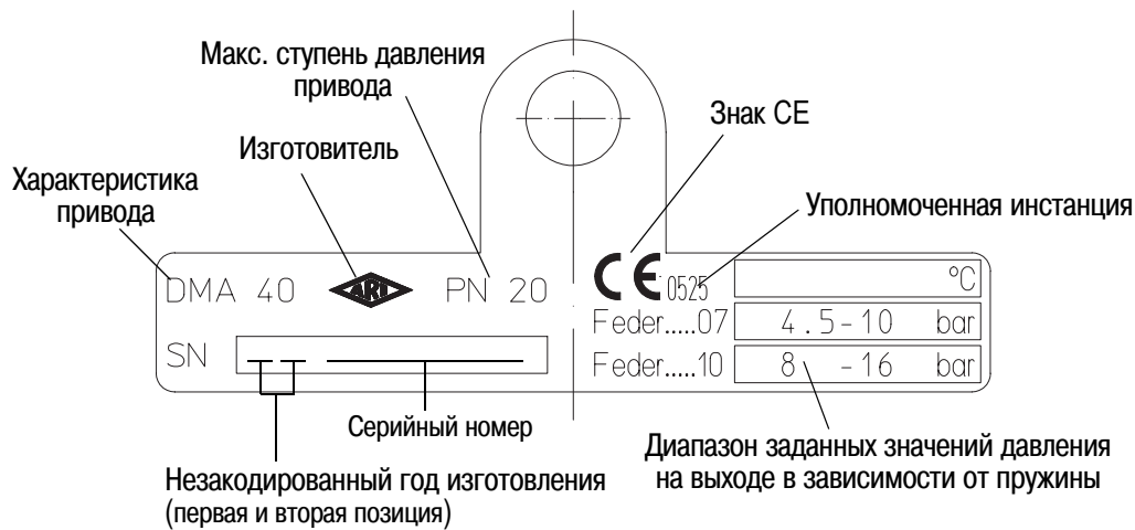
Рис. 3: Привод
