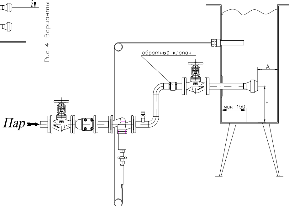
Рис 5 Схема монтажа при трубопроводе расположенном ниже уровня жидкости в резервуаре
