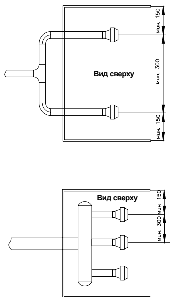
Рис 4 Варианты монтажа двух и трех инжекторов
